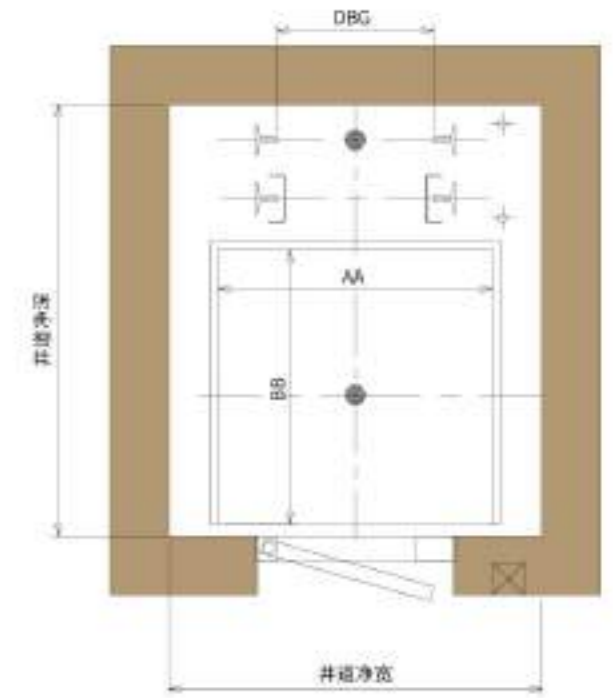
平面布置图
