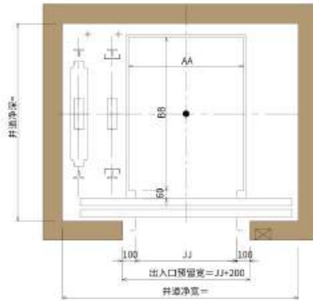
平面布置图 Layout plan
