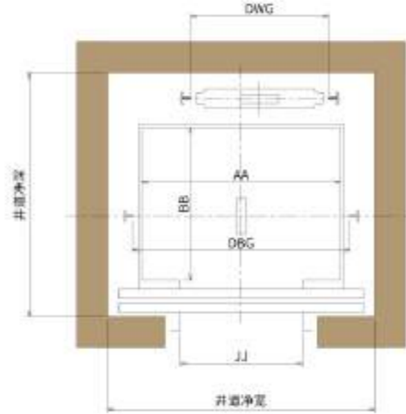
平面布置图 Layout plan
