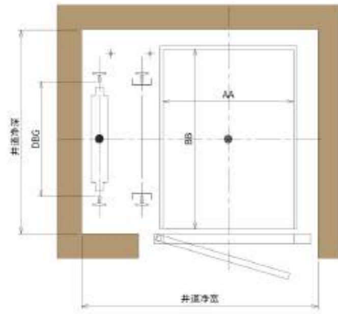
平面布置图 Layout plan
