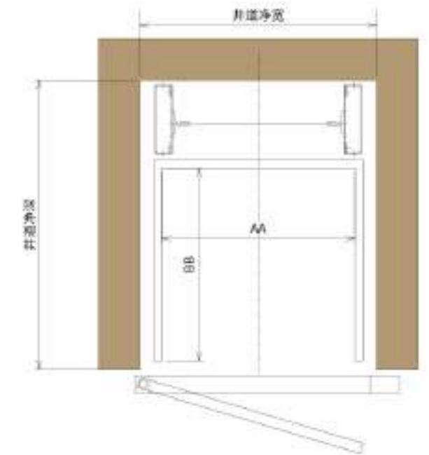
平面布置图
