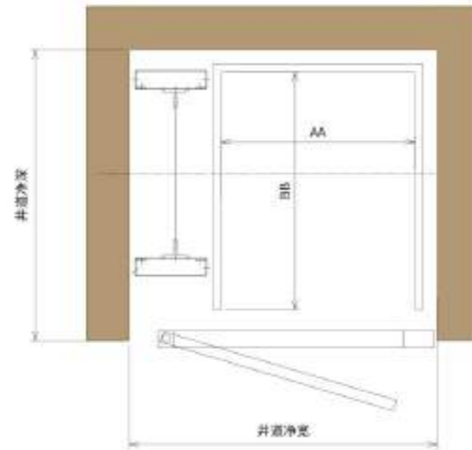
平面布置图
