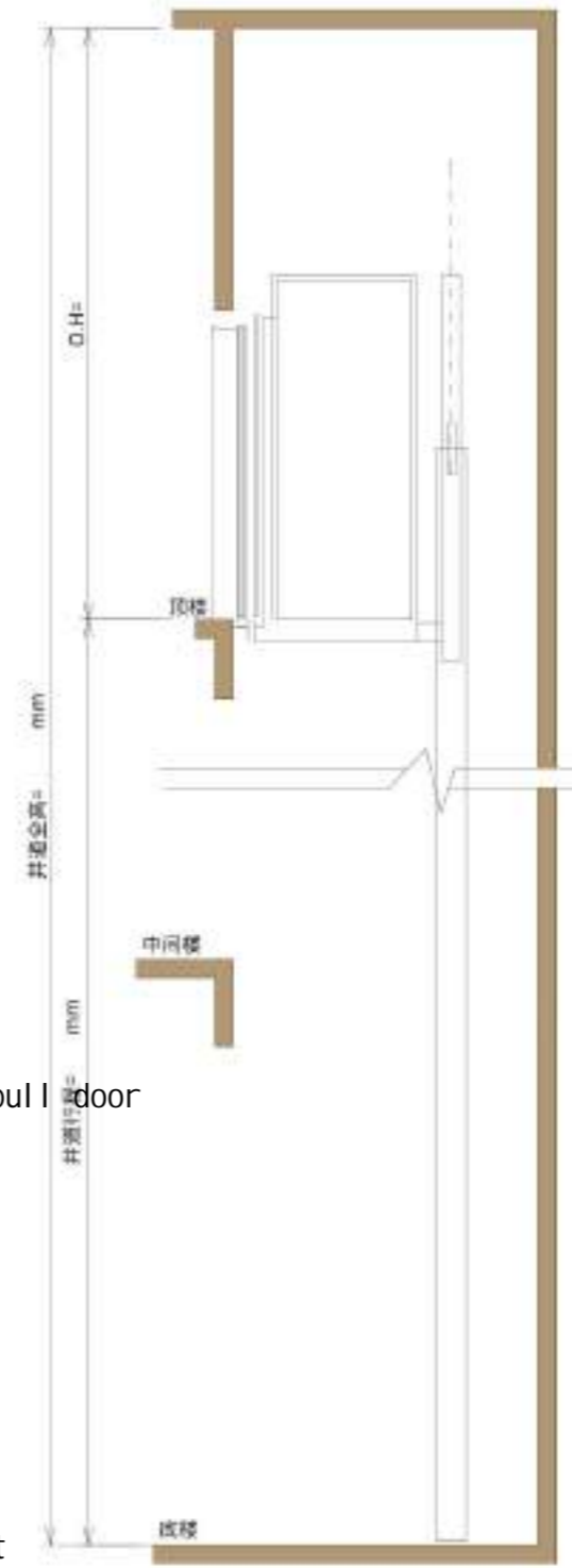
井道立面图
