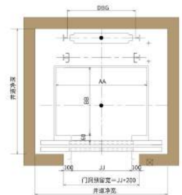
平面布置图
