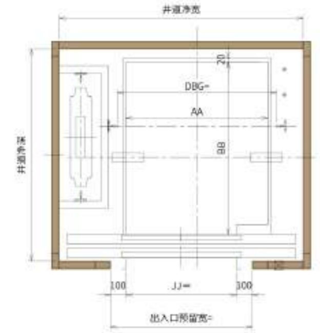
平面布置图
