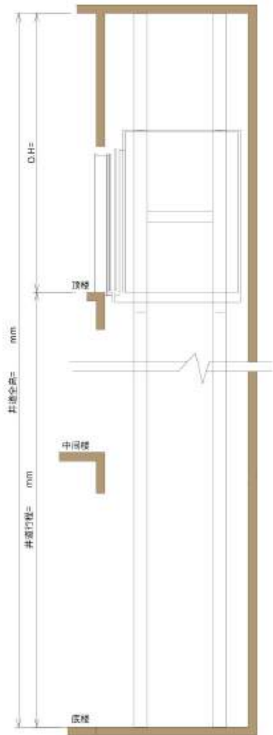
井道立面图
