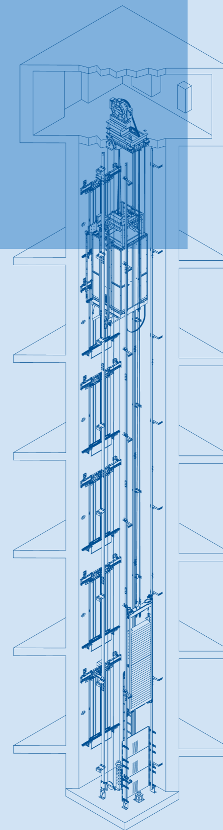
ШАХТА С МАШИННЫМ ПОМЕЩЕНИЕМ
