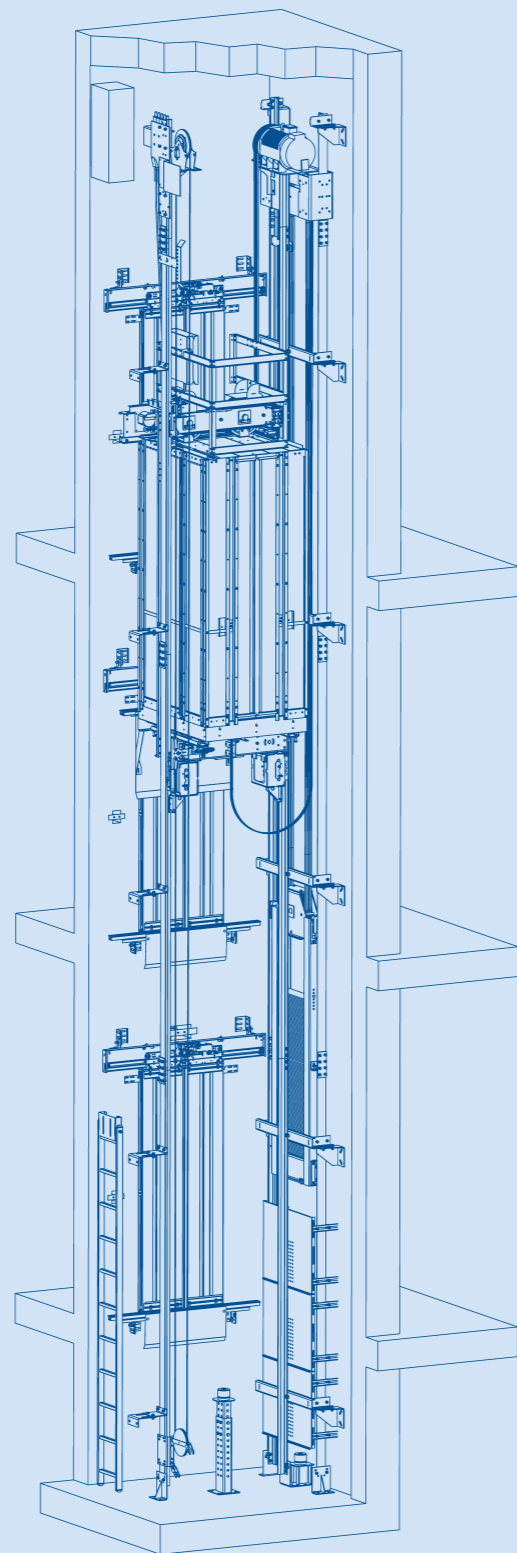
ШАХТА БЕЗ МАШИННОГО ПОМЕЩЕНИЯ
